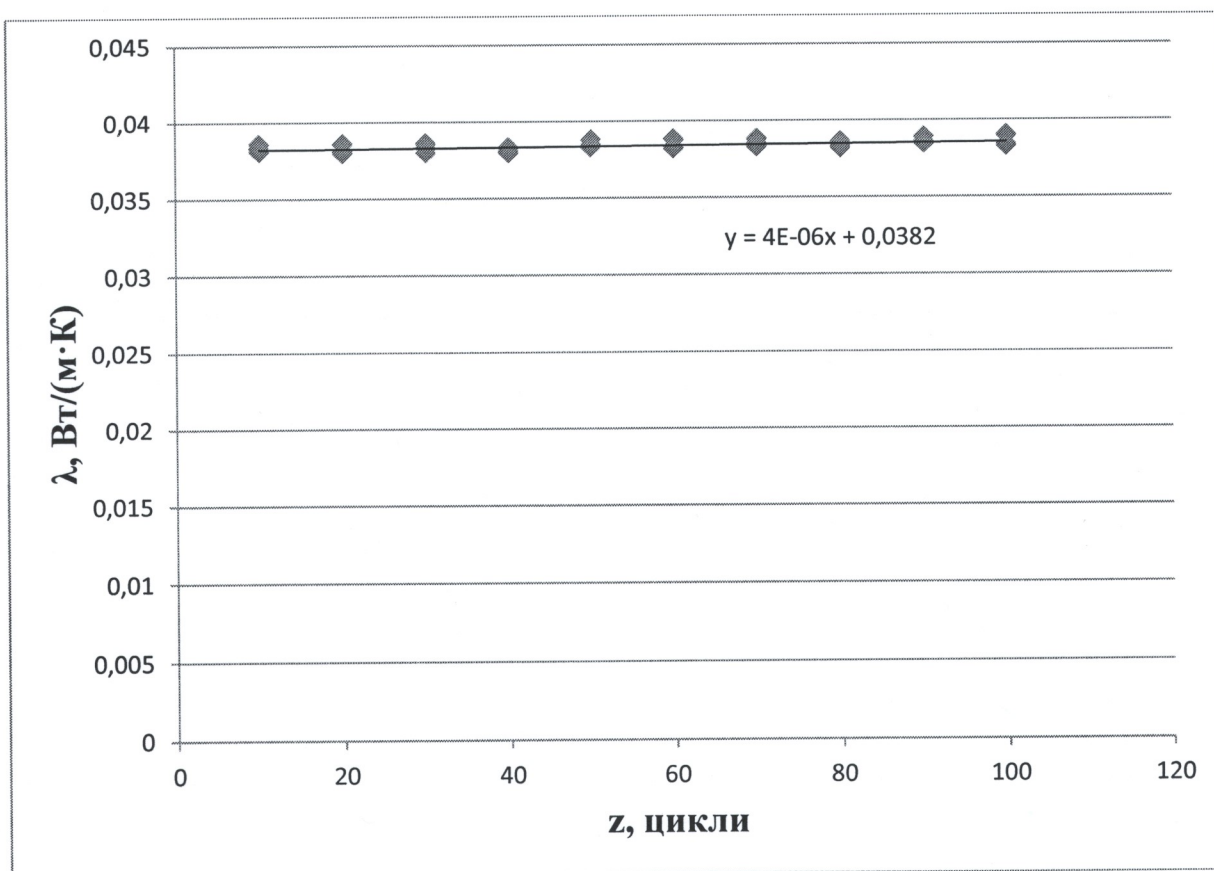
Рисунок 3 – Залежність теплопровідності від циклічних впливів
